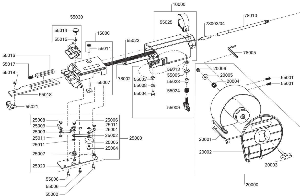
VORSATZ 3343 ATTACHEMENT 3343 SUPPORT CHARGEUR 3343
